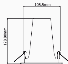
VISTA LATERAL
